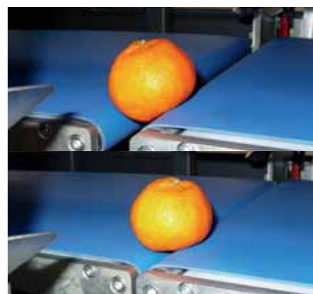
Tappeti avvicinati standard flessibilità nel range di prodotti. Permette di lavorare anche prodotti molto piccoli/tondi.
