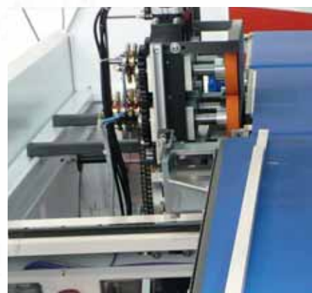
Ridotta distanza tra saldatore laterale e prodotto. Risparmio di 10 cm di film per ogni confezione.
