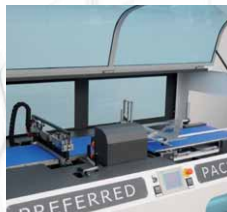
Macchina a saldatura laterale 3 nastri: flessibilità e risparmio.
