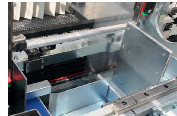
Particolare del raggruppatore sovrappositore. La versatilità permette veloci cambi "formato" per diverse composizioni. Detail of grouper staker. The flexibility allows fast change of format and different products composition.
