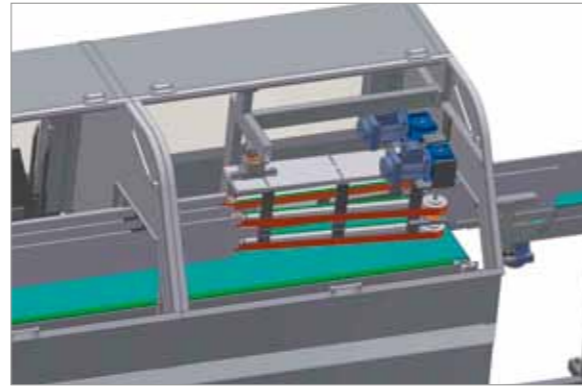
Deviatore automatico Automatic diverter
