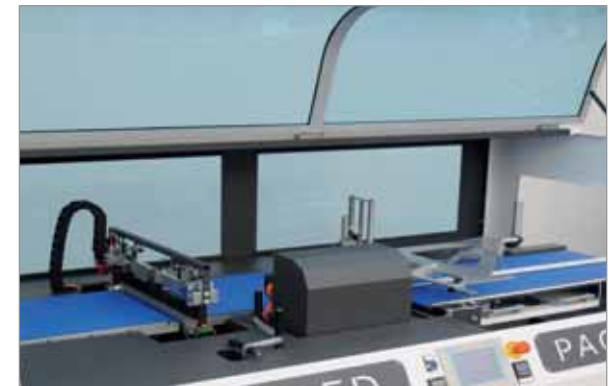
Sistema a saldatura laterale Side sealing machine
