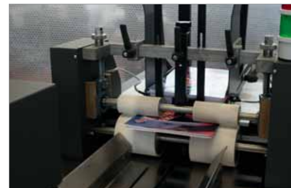
Sfilatore: per giornali, riviste o altri prodotti. Drawer Feeder: for magazines newspapers, books or other products.
