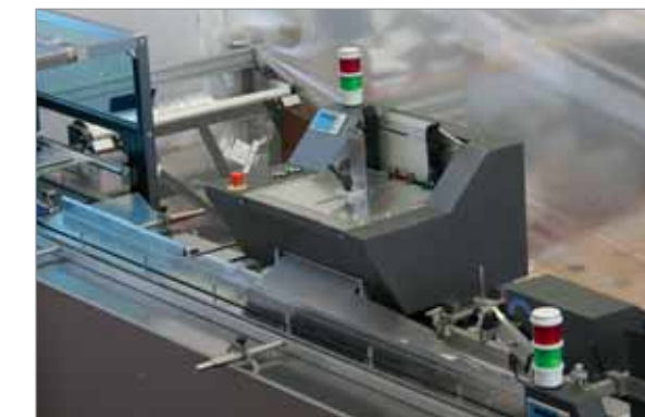
Nastro a palette: permette l'entrata in sicurezza dei prodotti in macchina anche ad alta velocità. Le palette spingono infatti il prodotto fino al nastro d'ingresso. Fully automatic packaging line for mailing and fast application Flighted Conveyor: for safe entrance of the products inside the machine.
